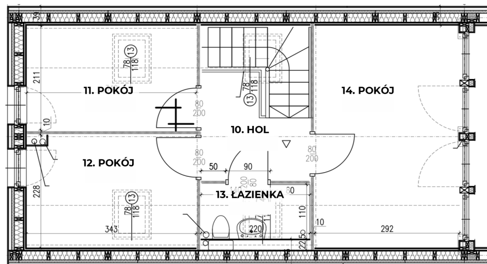
RZUTY
